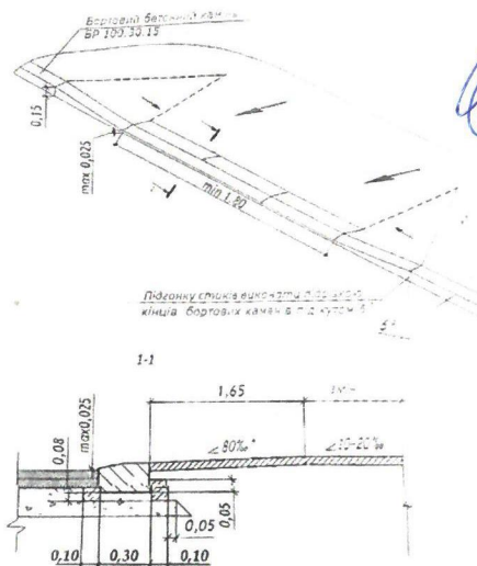
Типова схема влаштування понижених бордюрних каменів
